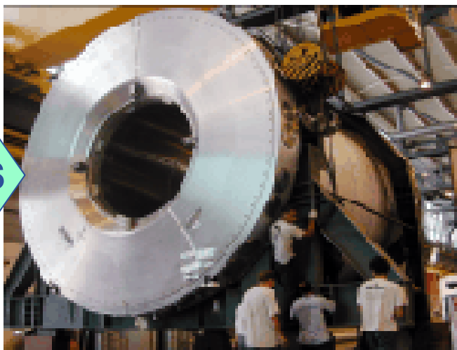
ATLAS
