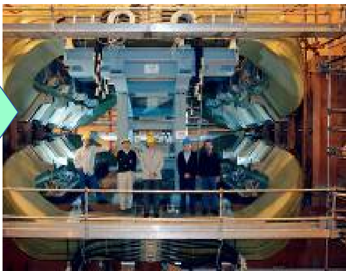
LHCb
