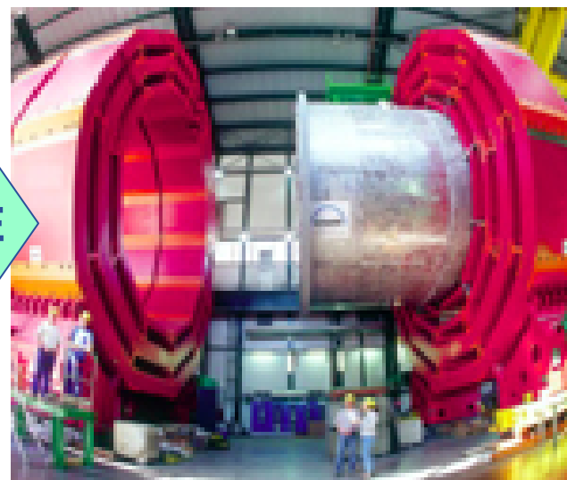
ALICE
